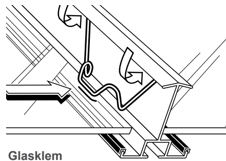
Glasklem
